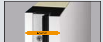
Thermisch getrenntes Türblatt
